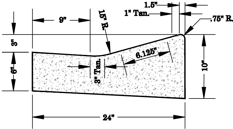
LIP CURB
